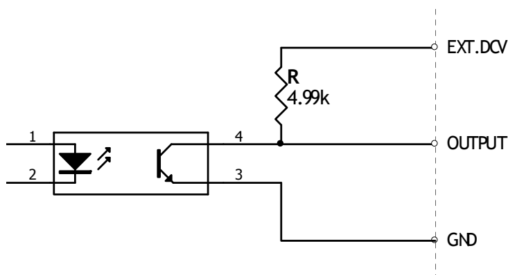
图 5-2 内部原理图
